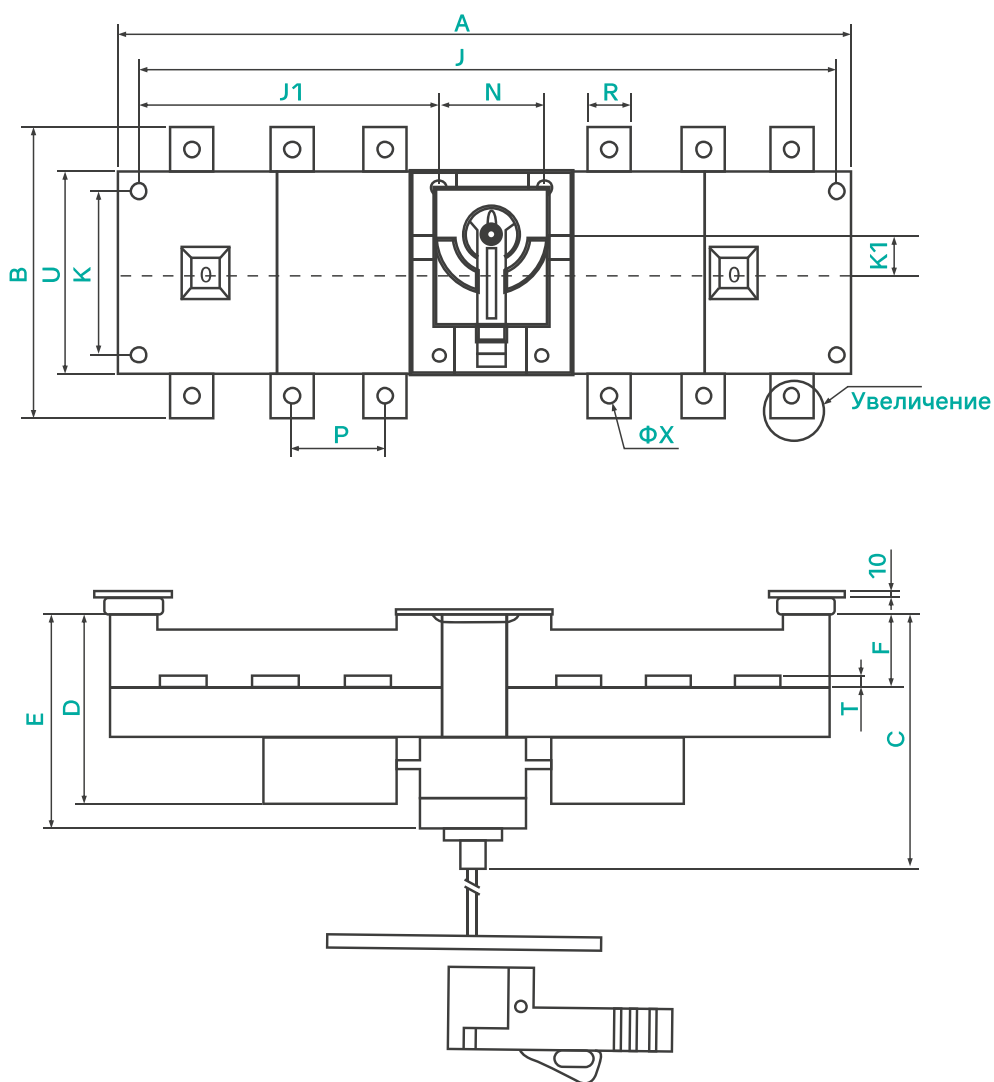
GLZ2-160A~1600A управление с дверцы шкафа
