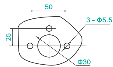
GL-1000~3150 Размеры монтажной панели ручки управления с дверцы шкафа
