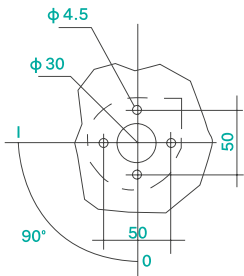
GL-125~630 размеры монтажной панели ручки управления с дверцы шкафа
