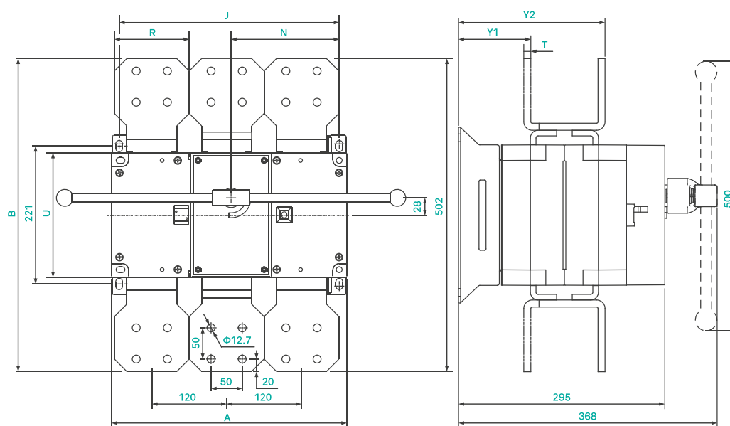
GL-3150 прямого управления
