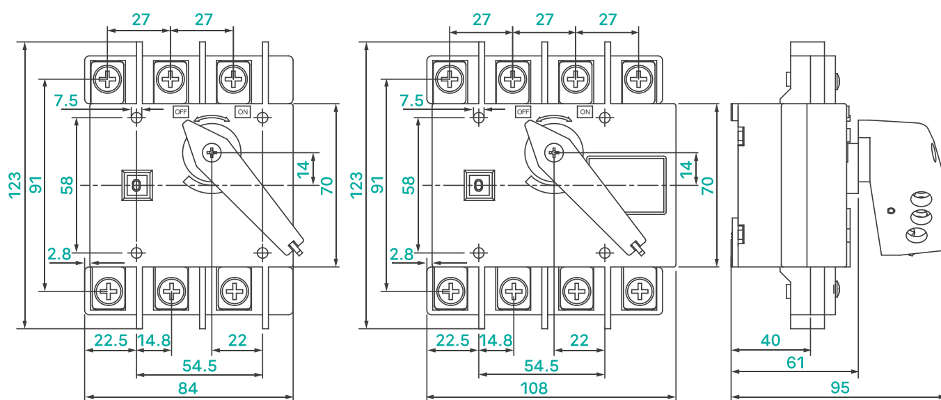
GL-100 прямого управления
