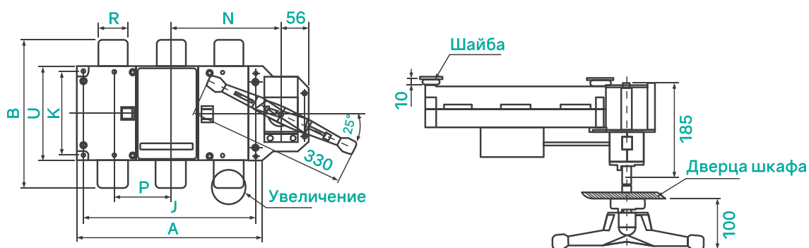
GLC-1600A/3 управление с дверцы шкафа
