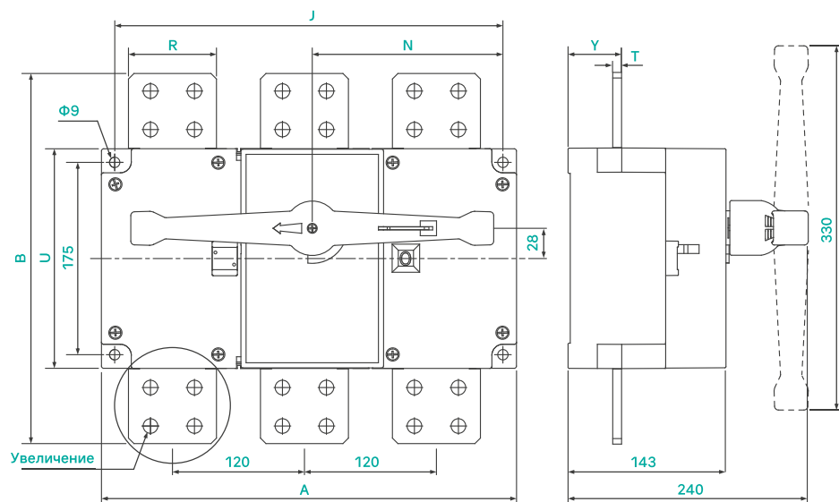
GL-1600 прямого управления
